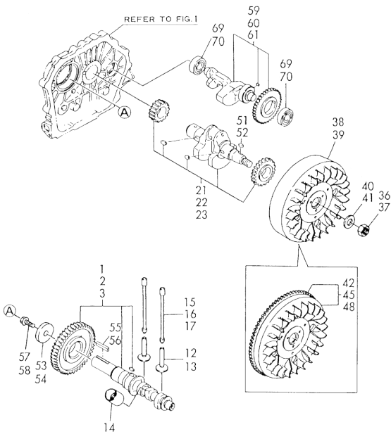
Fig.5. CAMSHAFT & CRANKSHAFT
