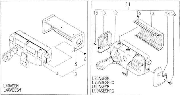
Fig.4. MUFFLER
